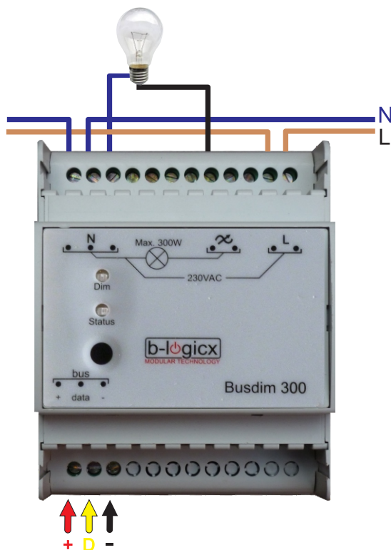
Aansluiting DIM-300-1K
