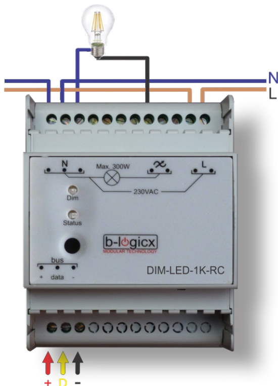
Aansluiting DIM-LED-1K-RC
