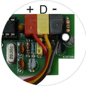
Aansluiting ASD-ART24
