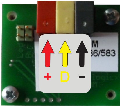
Aansluiting BDM-HYDRO
