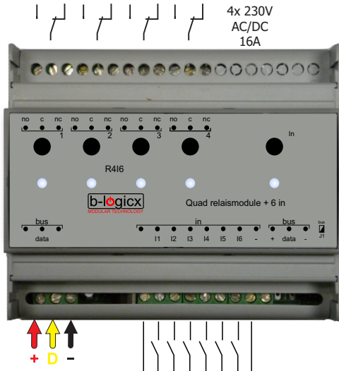
Aansluiting R416
