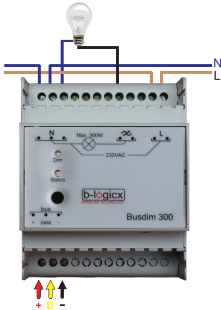
Aansluiting DIM-300-1K
