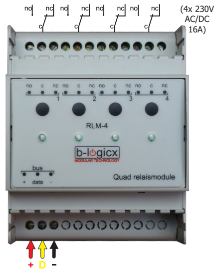
Aansluiting RLM-4
